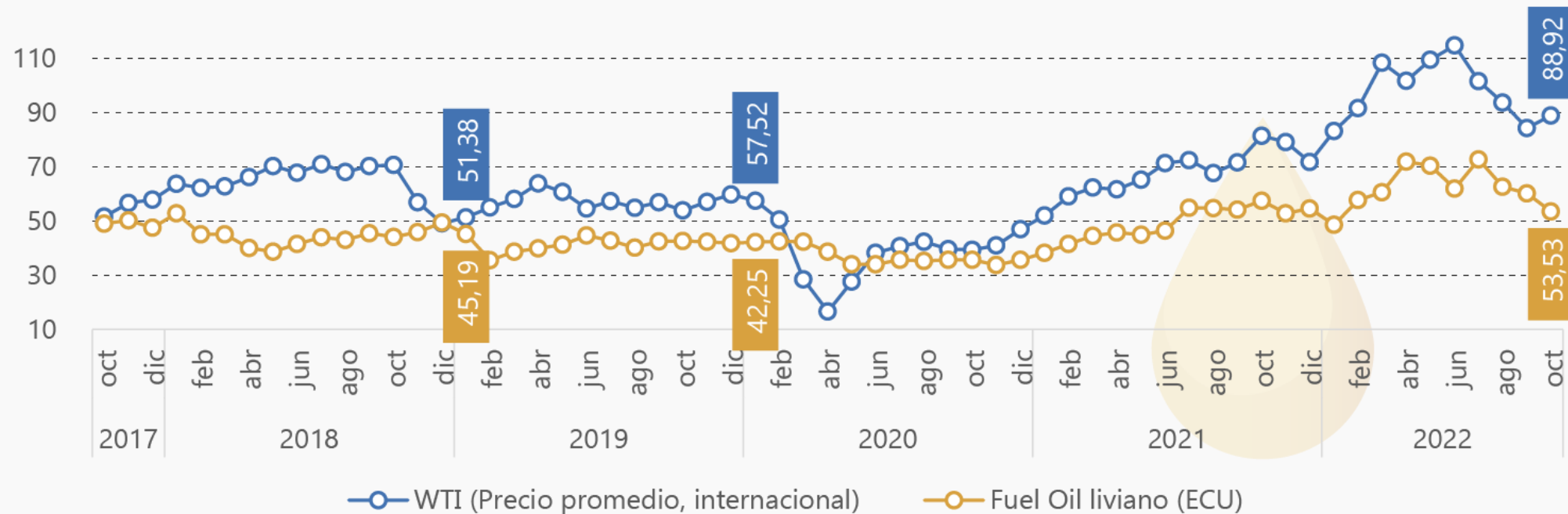
Cotización internacional del WTI versus Precio de comercialización de Fuel Oil Liviano (precio promedio para cada mes, dólares por barril)
